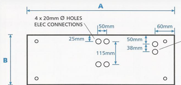
FELÜLNÉZET
