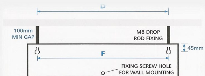
HÁTULNÉZET
